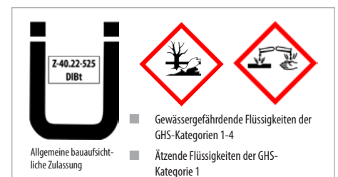
Wannerverbinder
